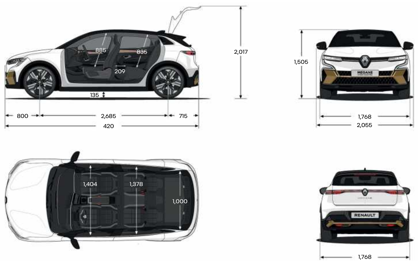
Dimenzije (mm)
