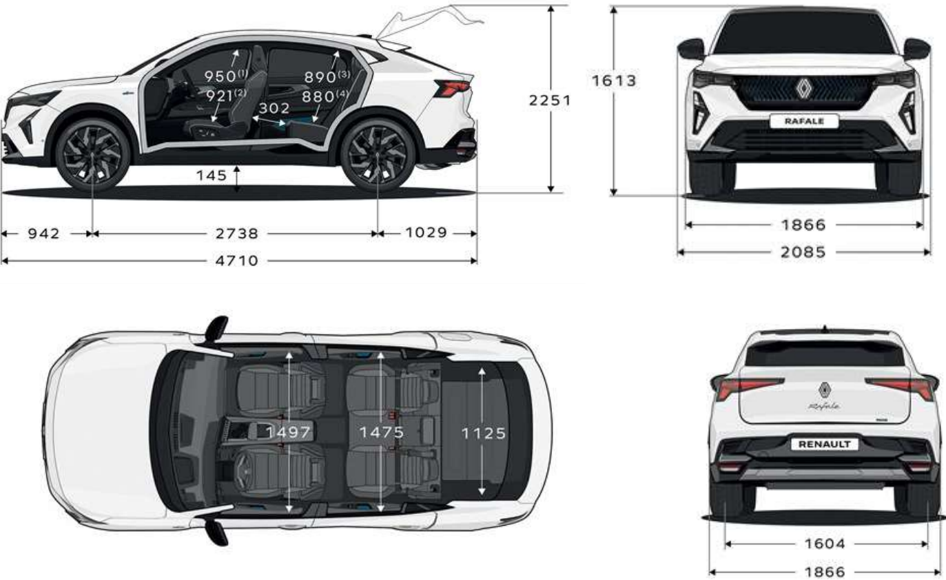
Dimenzije (mm).
