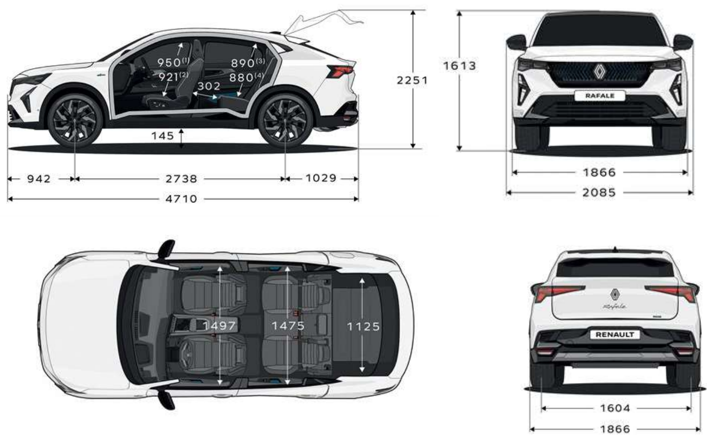
Dimenzije (mm).
