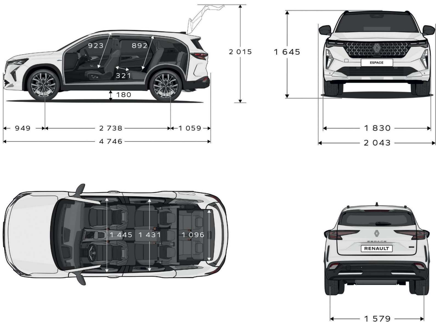
Dimenzije (mm).
